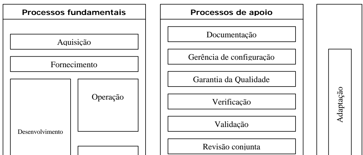
Figura 2- Processos de Ciclo de Vida do Software [ISO12207: 97].
